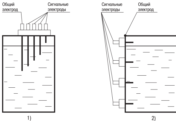
Рисунок 6.2 – Установка кондуктометрических датчиков
